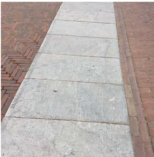
rand rondom Heuvel (40 cm) gelijke hoogte klinkerverharding of licht oplopend, hardsteen (OF hergebruik bestaande banden)
